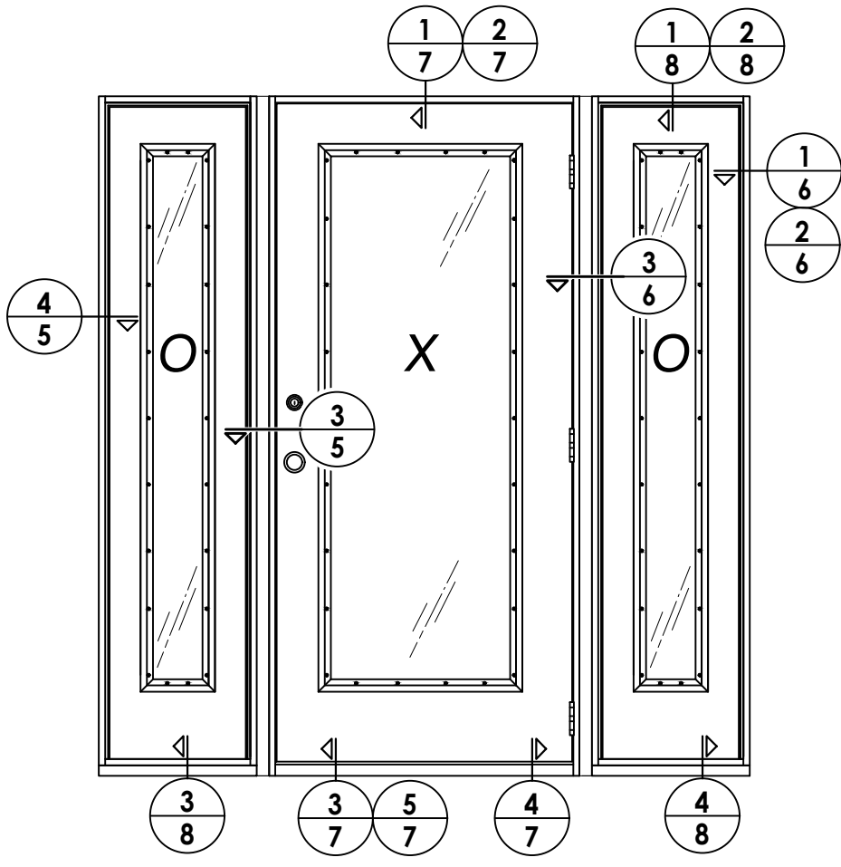
ELEVATION (OXO)
